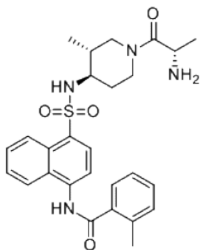
PC-6197901, DMSO-d6
